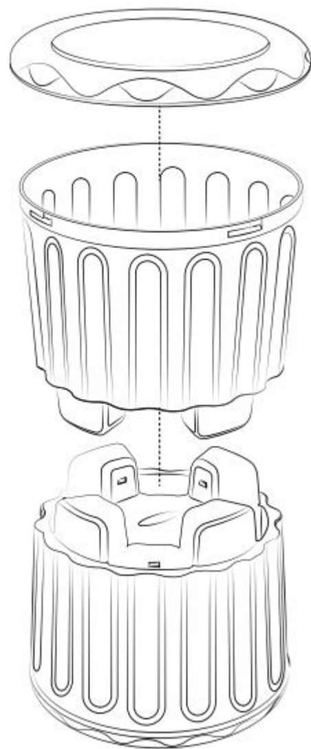
拼接方法示意图 Assembly diagram
