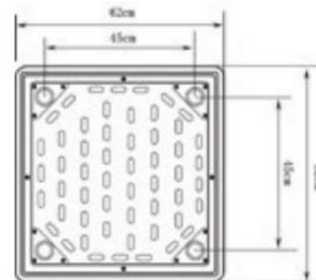
桌面安装示意图 Tabletop installation
